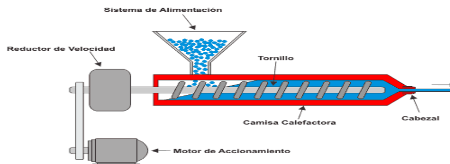
Figura 3. Proceso de extrusión (Modelo)
