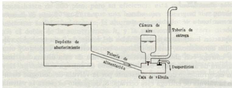
Figura 4. Esquema sistema de ariete.
